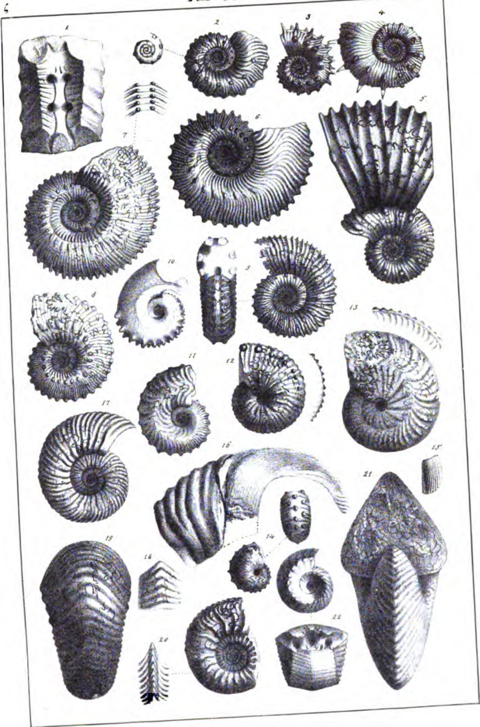
Guenstedt, Jura.
